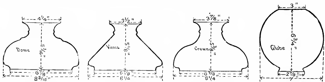
Fig. 3426. "DOME" LAMP-SHADE. Fig. 3427. "VIENNA" LAMP-SHADE. Fig. 3428. "CROWN" LAMP-SHADE. Fig. 3429. "GLOBE" LAMP-SHADE OR LAMP-GLOBE.
